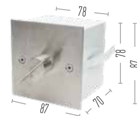
Luftklappengriff quadratisch, Aufputz – Design 3
