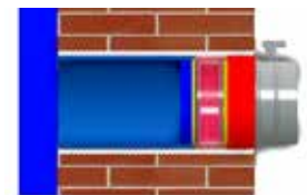
mit Rohrdämmmatte
