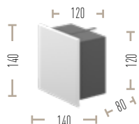
PutzkapSEL quadratisch, weiß – Aufputz
